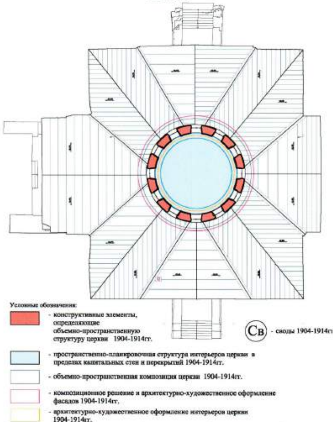
Схема предмета охраны План барабана
