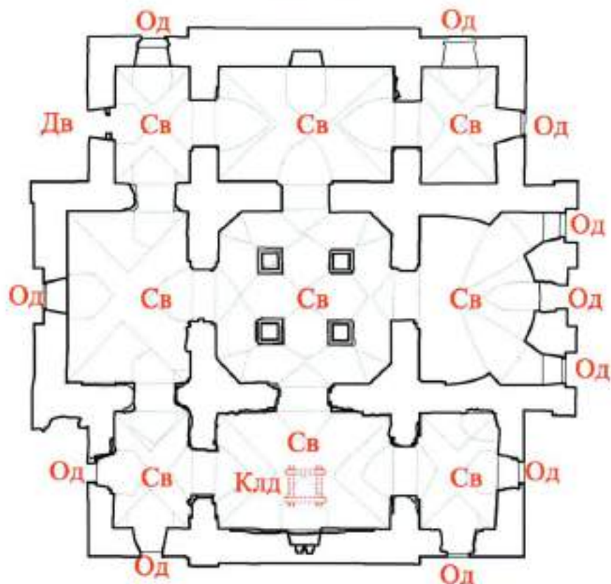
Схема предмета охраны План подвала
